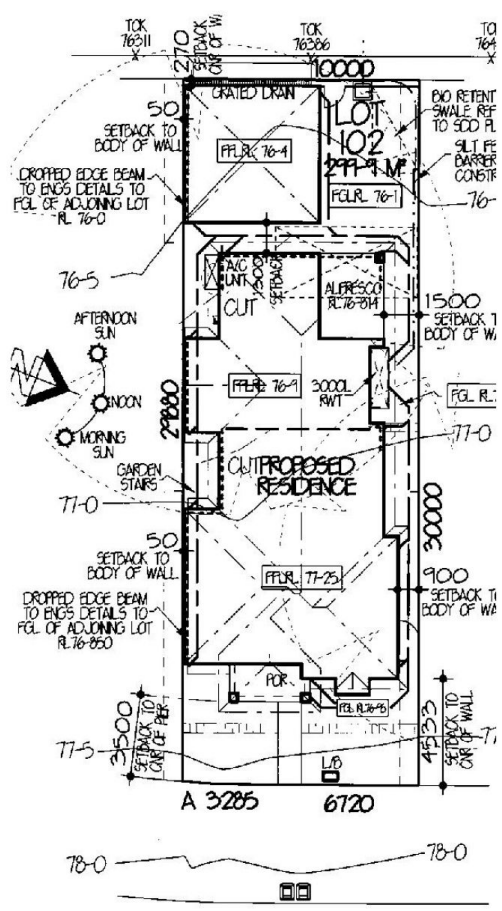
HAZLETT ROAD SITE PLAN 1:200
